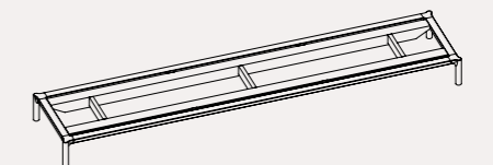
0,5 MODULE 400/150/470 mm
